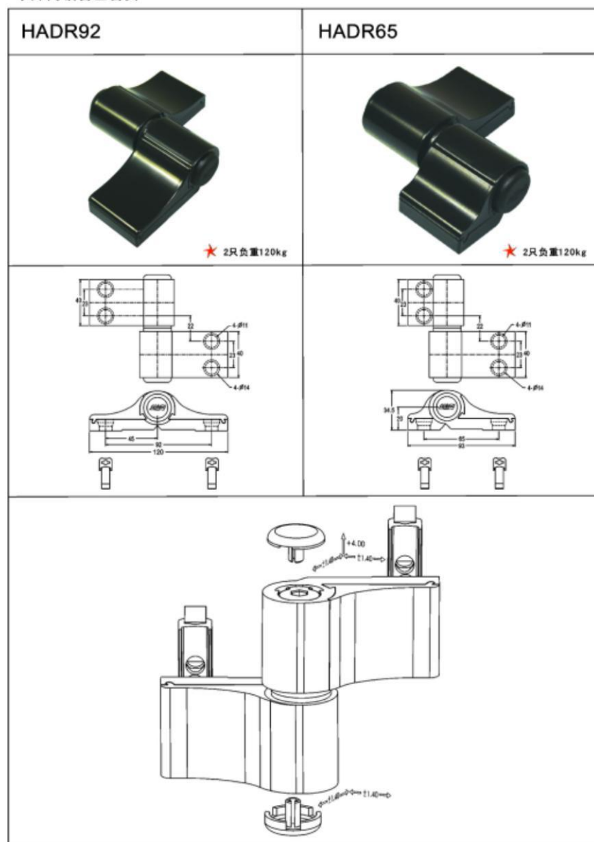
平开门铝合金合页
