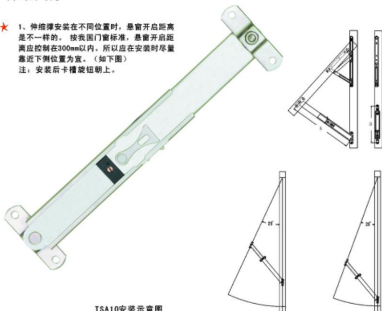
TSA10安装示意图
