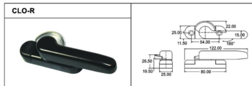
月牙锁钢扣 (有多款尺寸可供选择)
