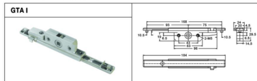
配合内平开下悬窗用传动盒
