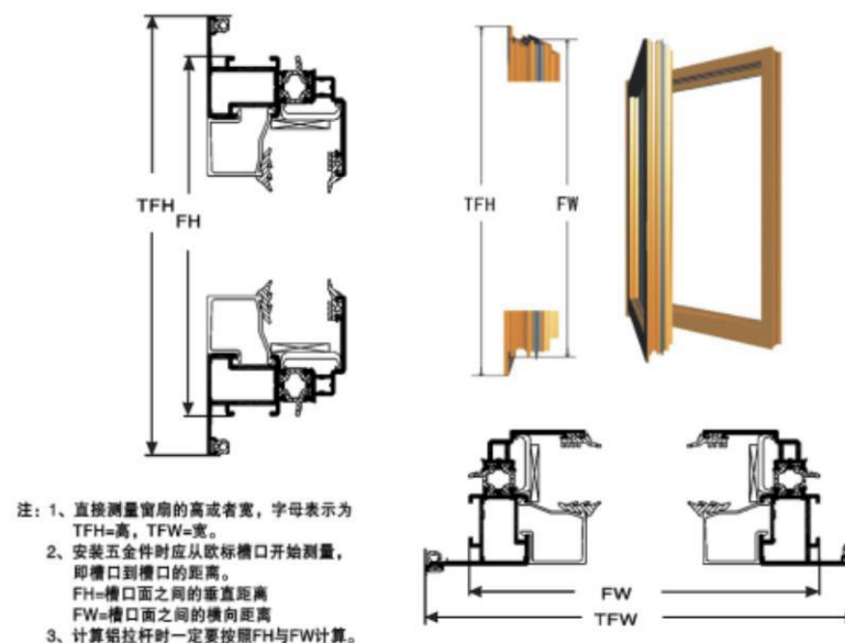
FW和FH的说明
