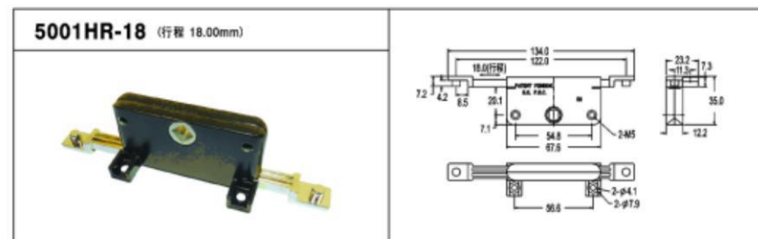
配合方轴多点锁使用的多款双向传动盒
