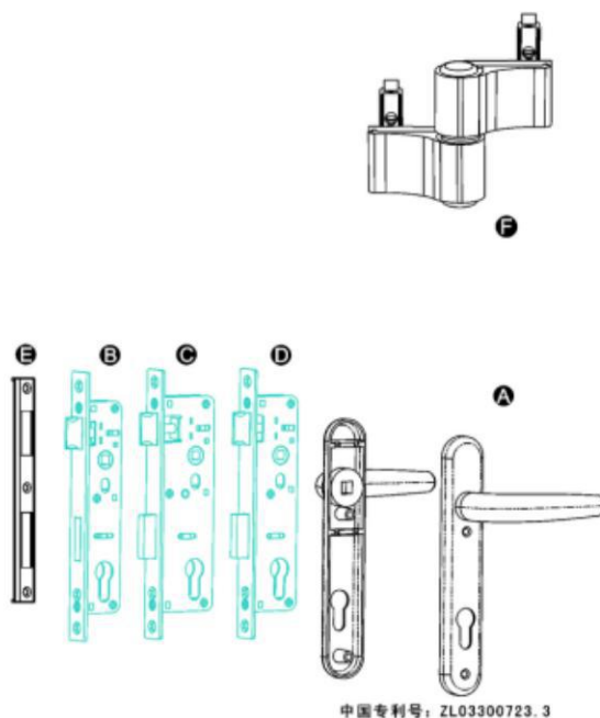
B HDLS18.5-7 锁盒
