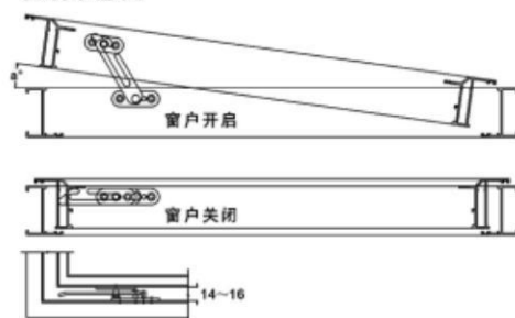
安装示意图
