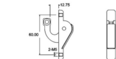
DBM-UP 上拉锁
