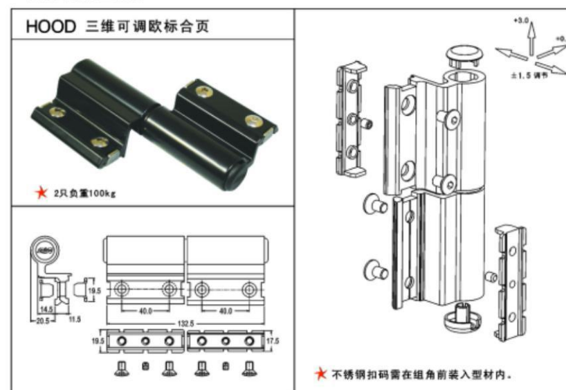
平开门锌合金合页
