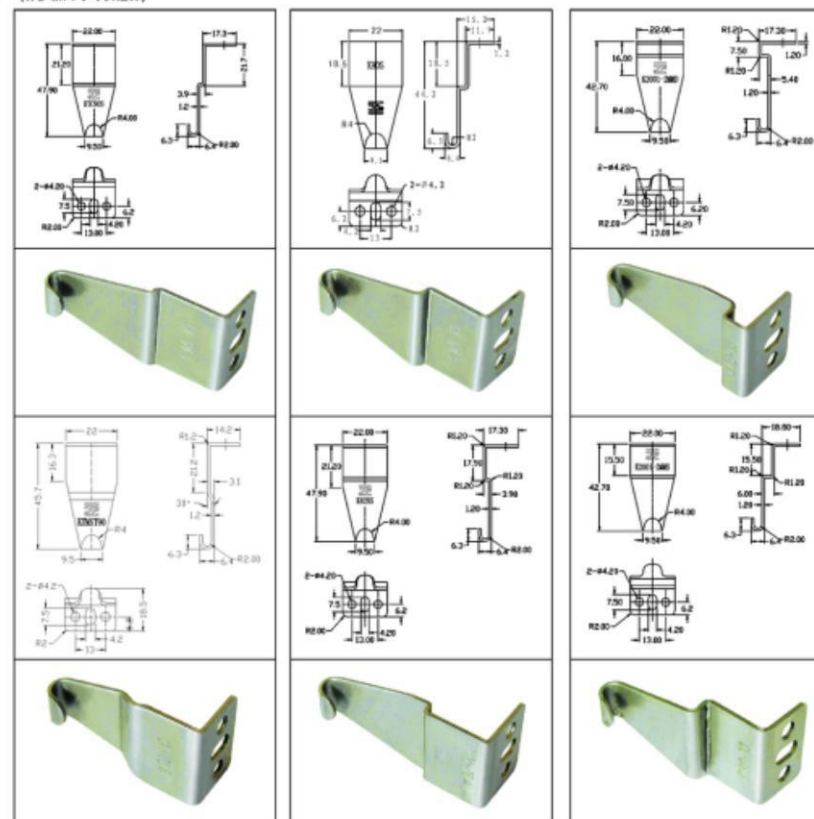
月牙锁钢扣 (有多款尺寸可供选择)
