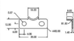
KXLS-S 上下执手用拉巴螺栓
