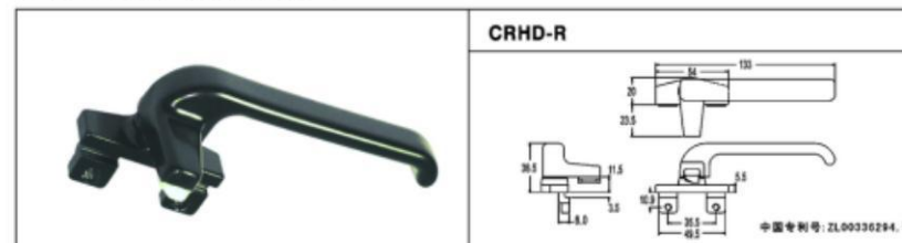
座脚七字执手-分离尼龙锁垫
