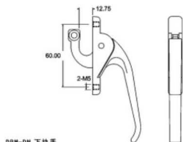
DBM-DN 下执手
