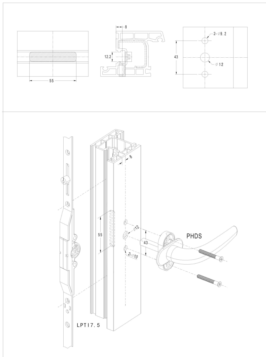
LPT17.5传动器开孔尺寸图
