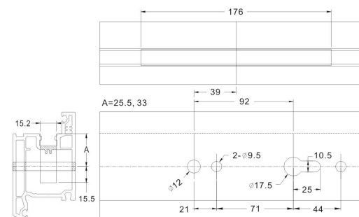
PHDLS44 锁盒开孔尺寸图
