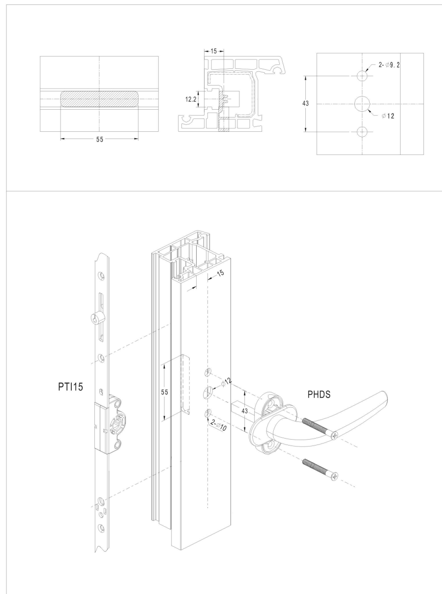
PTI15 传动器开孔尺寸图
