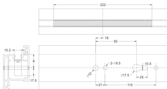
PHDLC30-8 锁盒开孔尺寸图
