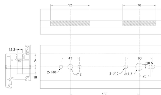
PGBK30 传动盒开孔尺寸图
