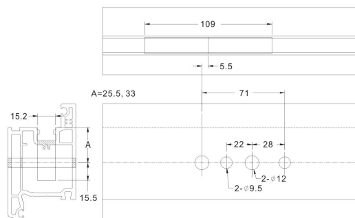
PHDLP44 锁盒开孔尺寸图
