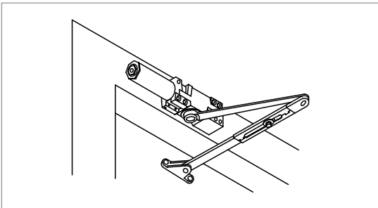
门框安装
