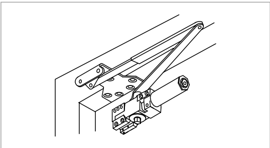
平行安装
