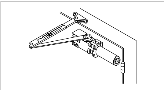
标准安装
