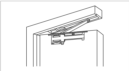
隐藏式安装
