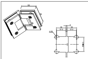
SH05 135°玻璃对玻璃浴室门夹
