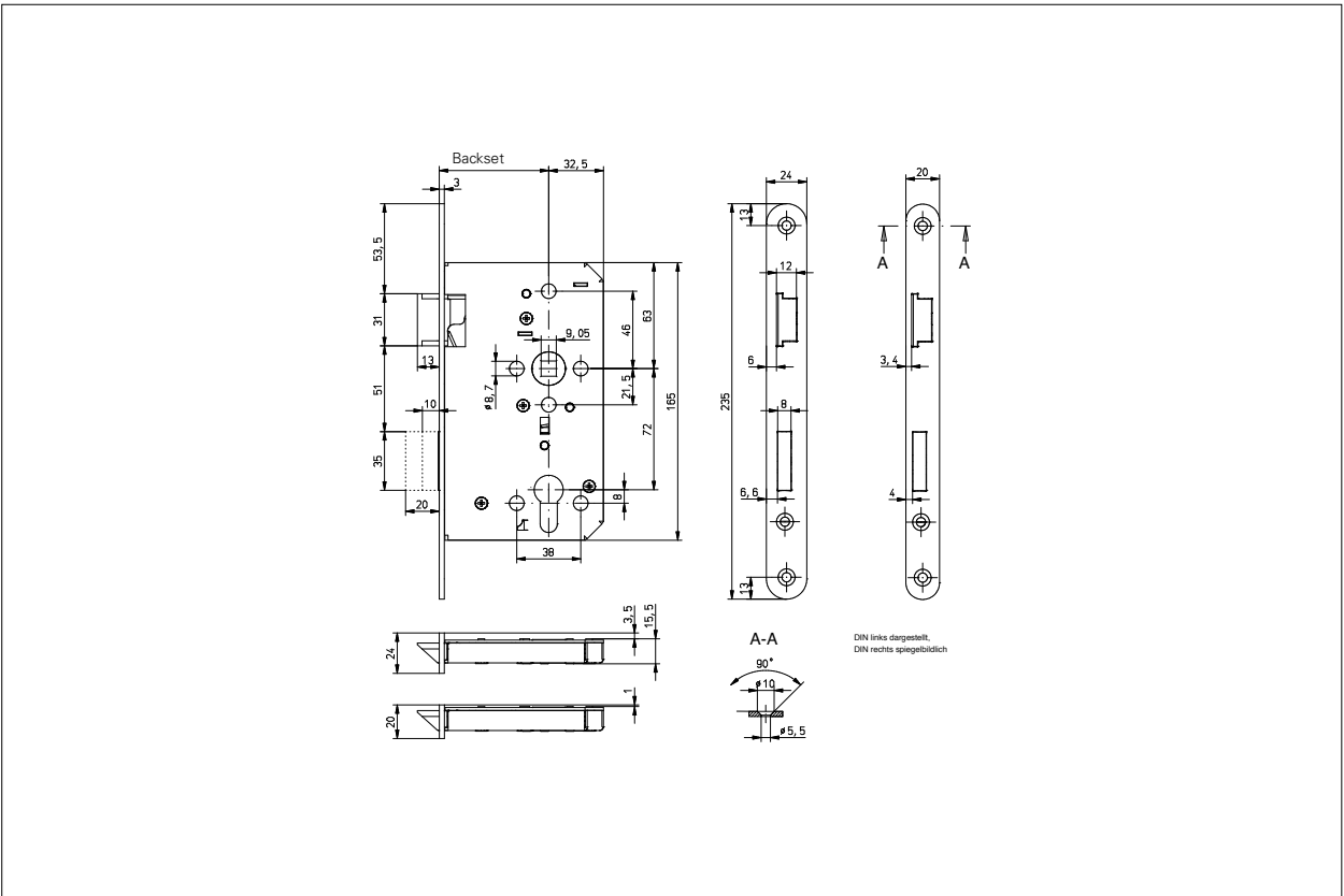
尺寸：GBS 81 防火标准锁
