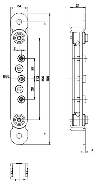
产品尺寸图
