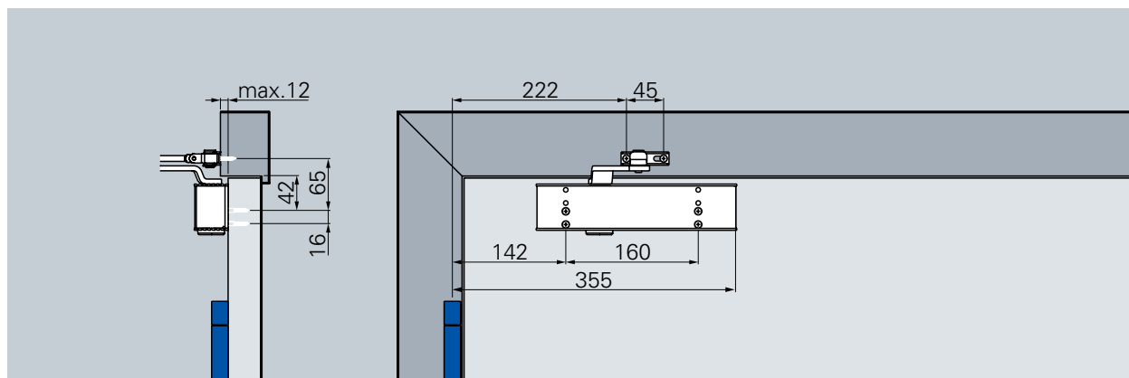
标准安装，铰链侧（可选DIN标开孔安装背板）
