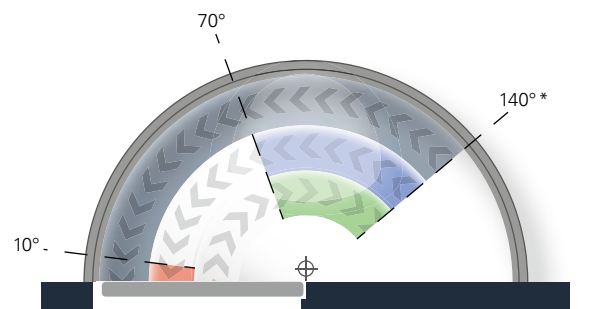
关门力度图示 ECO Newton TS-61, 铰链背侧
