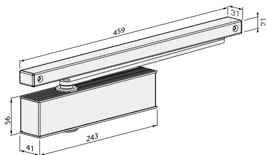
尺寸: TS-41带滑轨 B 可选
