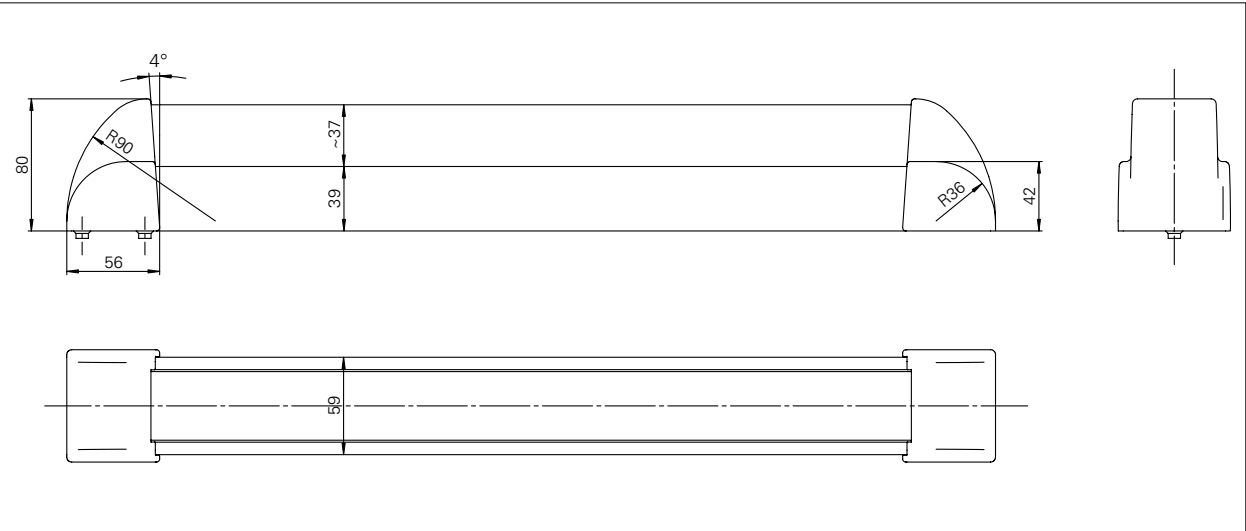
尺寸：EPN 2000 II
