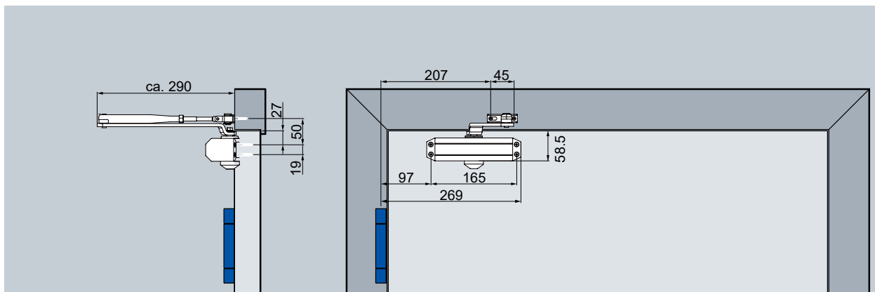
标准安装, 铰链侧
