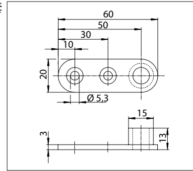
尺寸：联动式销杆门扇下置式导向套
