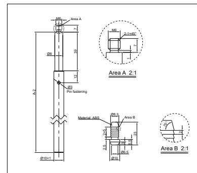
尺寸：门扇上置式联动销杆
