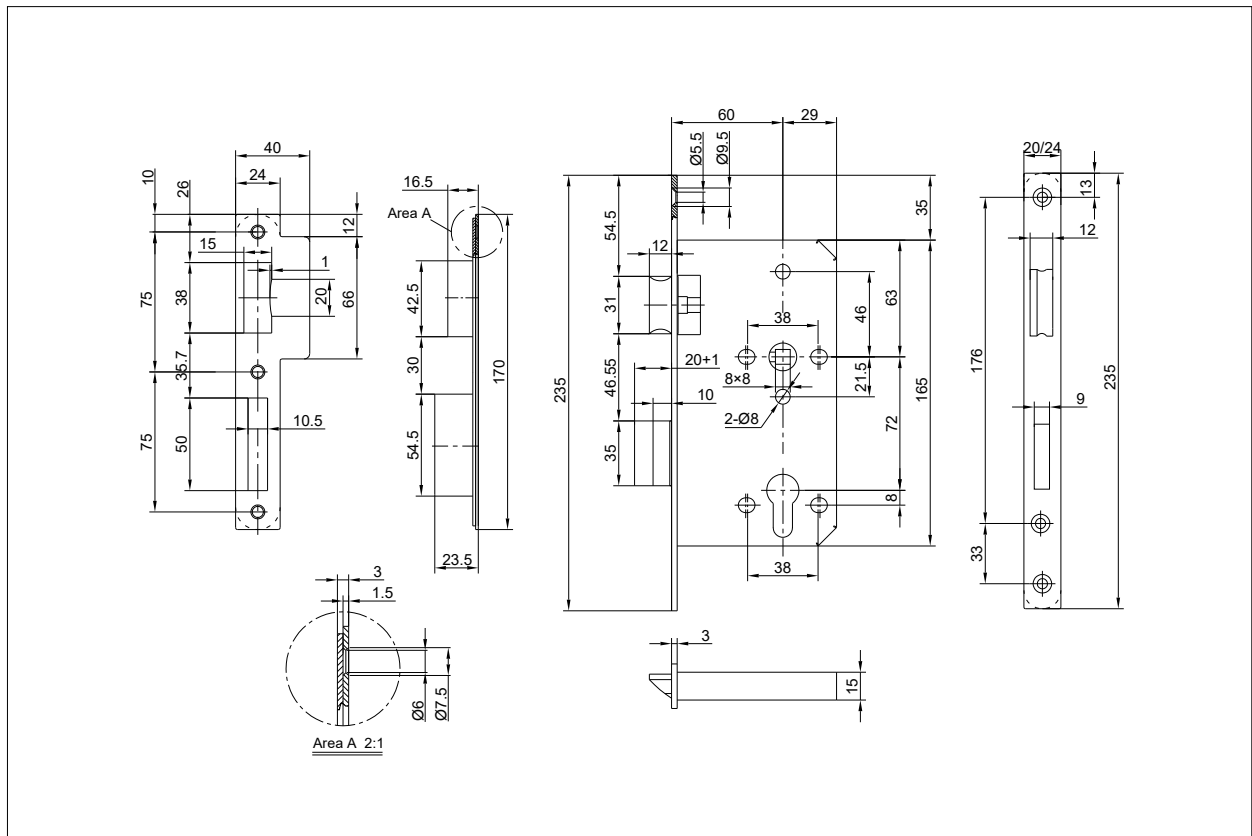
尺寸图：GBS 31 F SH 钢木门标准锁
