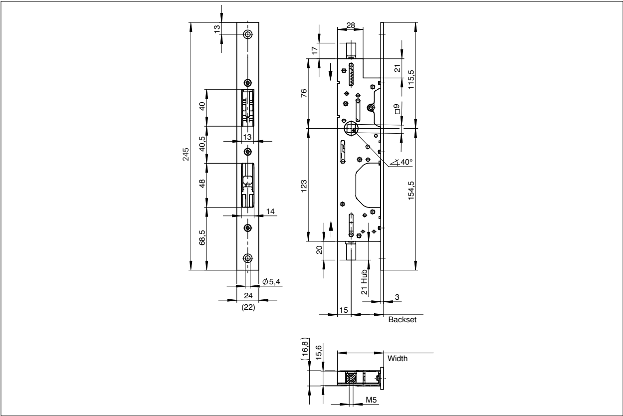
尺寸：GBS 98 双开型材门常闭扇防火逃生门插芯锁
