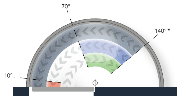
关门力度图示 ECO Newton TS-62, 铰链背侧
