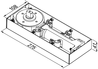
尺寸: FH 650
