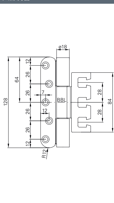
产品尺寸图
