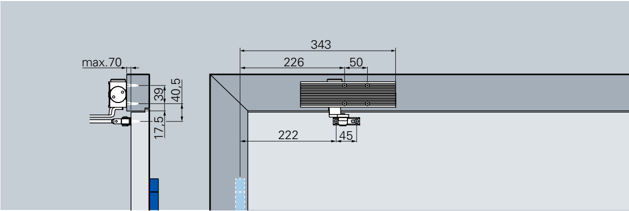
顶部安装, 铰链背侧 (EN 5)
