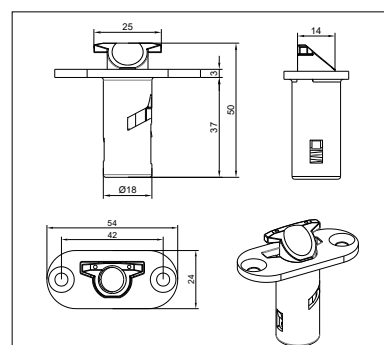
尺寸: ECO 171
