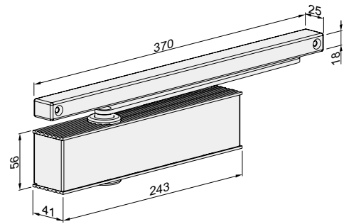
尺寸: TS-33 滑轨K
