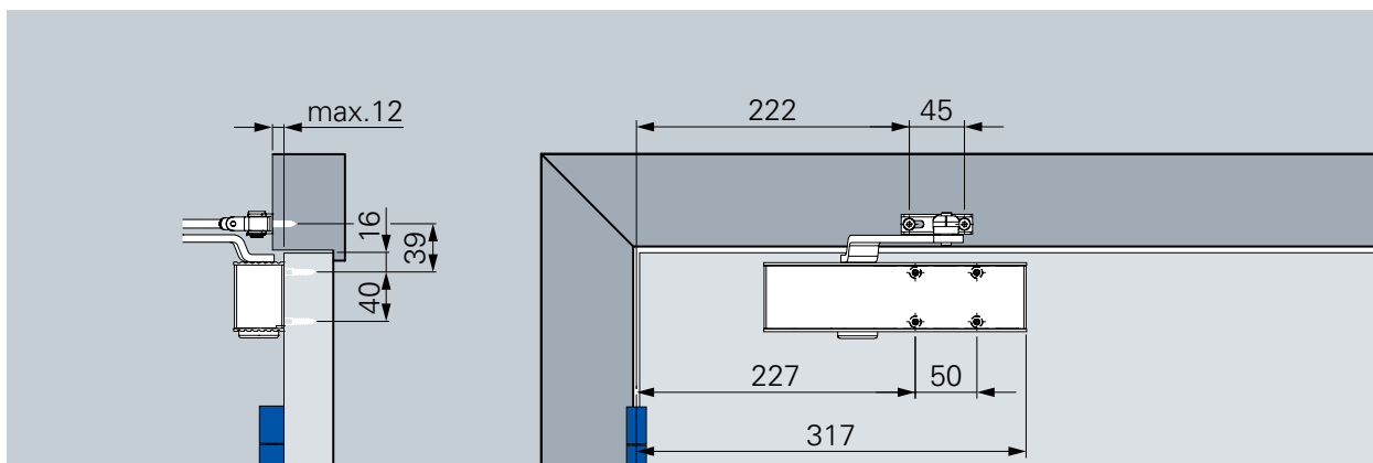
标准安装, 铰链侧 (EN 3),带安装版
