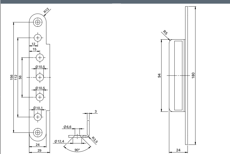
产品尺寸图
