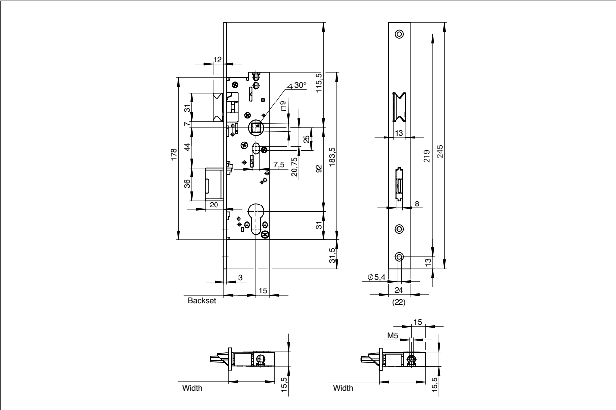
尺寸：GBS 97 双开型材门常开扇防火逃生门插芯锁
