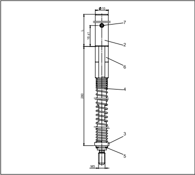
尺寸：门扇上置式联动销杆 GBS130/140
