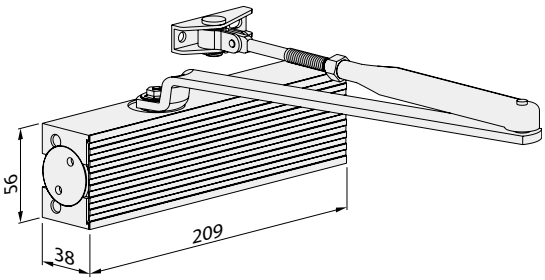
尺寸: TS-14
