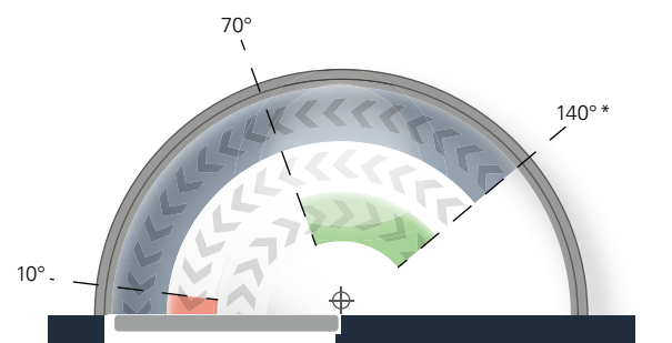
关门力度图示 ECO Newton TS-41, 铰链背侧
