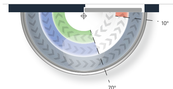
关门力度图示 ECO Newton TS-61，铰链侧
