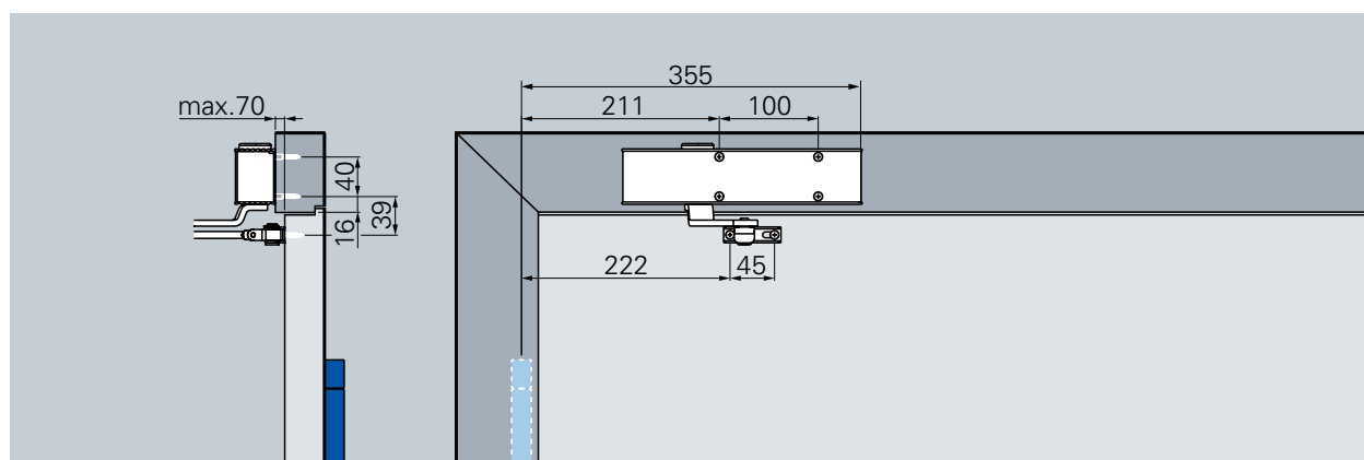
顶部安装，铰链背侧（闭门器直接安装，不带安装背板）
