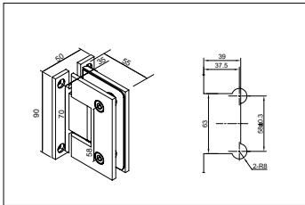
SH02 90°玻璃对墙浴室门夹 (分叉底板)
