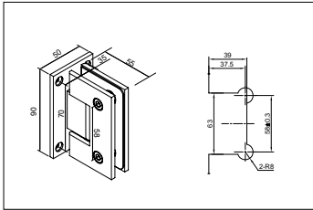
SH01 90°玻璃对墙浴室门夹 (标准底板)
