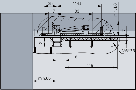
固定框架，顶部安装
