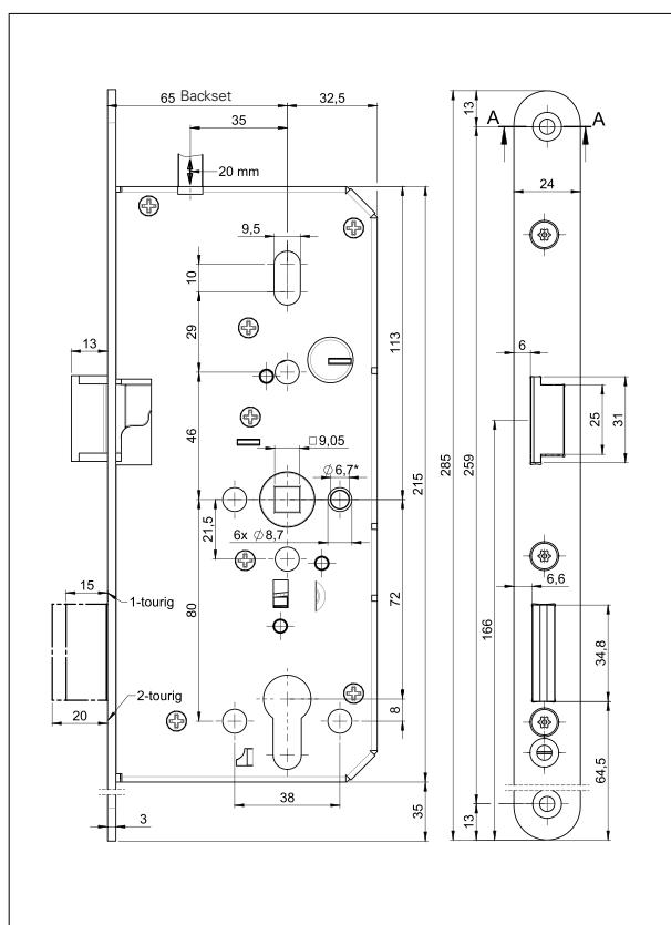
尺寸: GBS 130 防火插芯锁
