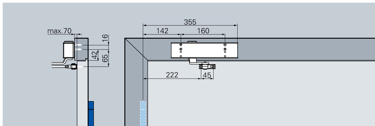
顶部安装，铰链背侧（可选DIN标开孔安装背板）
