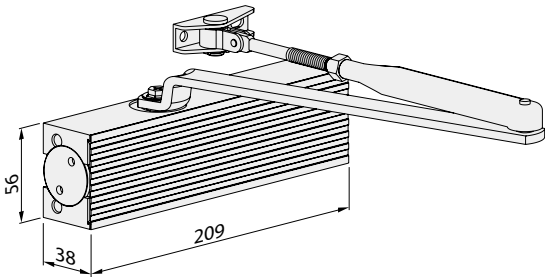
尺寸: TS-15
