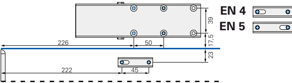
关门力度级别EN 4/5
