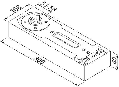
尺寸: FH 840
