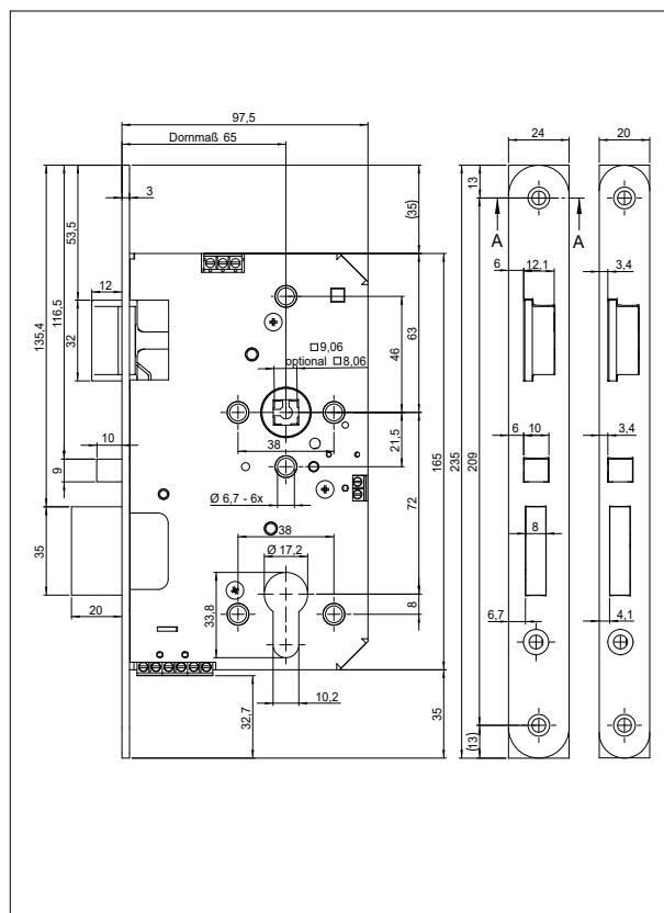
尺寸：GBS 90 防火逃生插芯锁体
