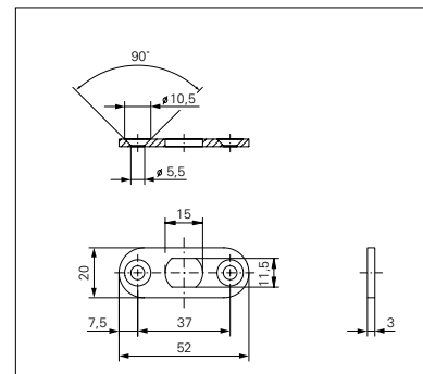
尺寸：门框下边沿锁挡片
