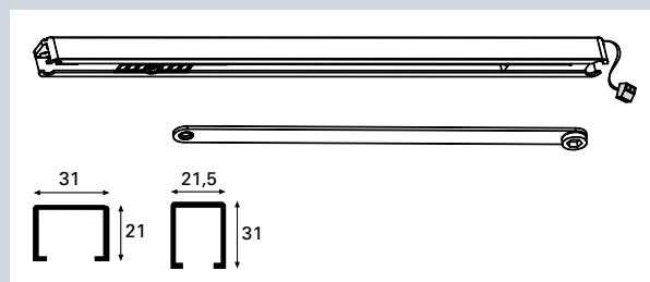
安装 滑轨 ITS-EF
