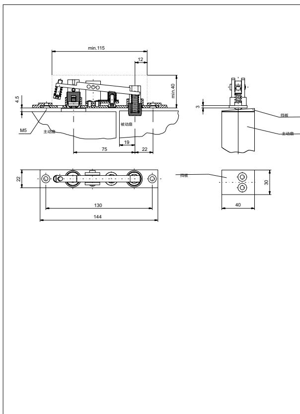
尺寸：碰珠斜舌型叠式锁系统
