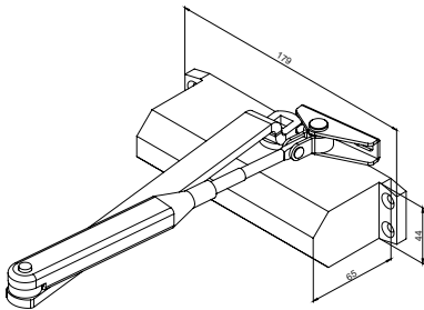
尺寸: TS-10
