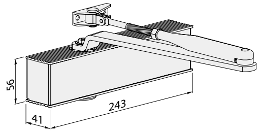
尺寸: TS-50
