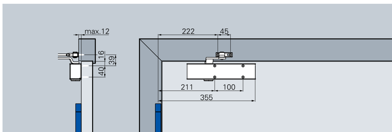
标准安装，铰链侧（闭门器直接安装，不带安装背板）
