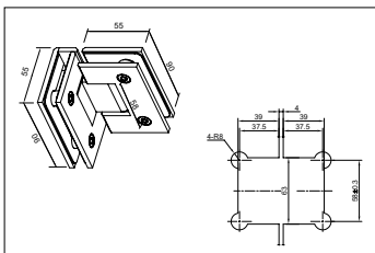
SH04 90°玻璃对玻璃浴室门夹
