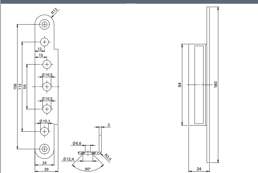
产品尺寸图
