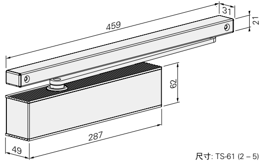
尺寸: TS-61 (2-5)
