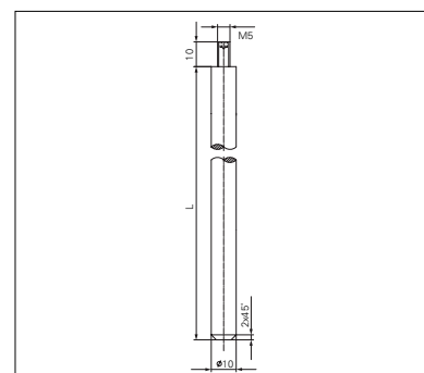
尺寸：门扇下置式联动销杆
