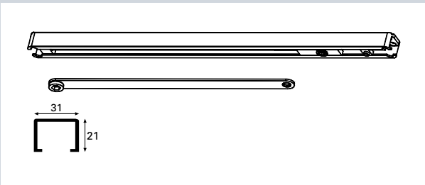
安装 滑轨 ITS-MFA
