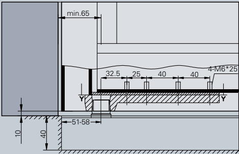
底部安装
