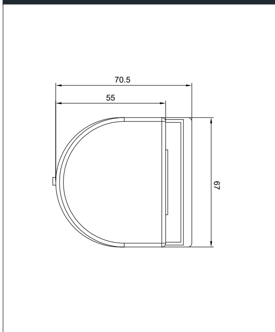
产品尺寸图
