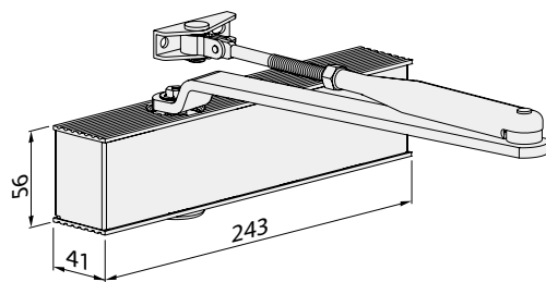
尺寸: TS-20
