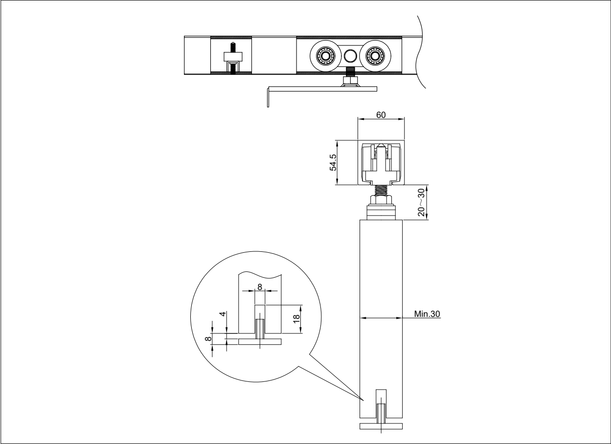
HR SL 160-W 木质推拉门示意图
