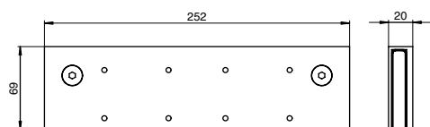
玻璃门夹配ECO牛顿 TS-41, TS-31, TS-50, TS-20
