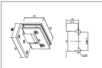
SH03 90°玻璃对墙浴室门夹 (偏心底板)
