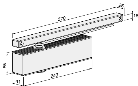
尺寸: TS-41带滑轨 K 标准
