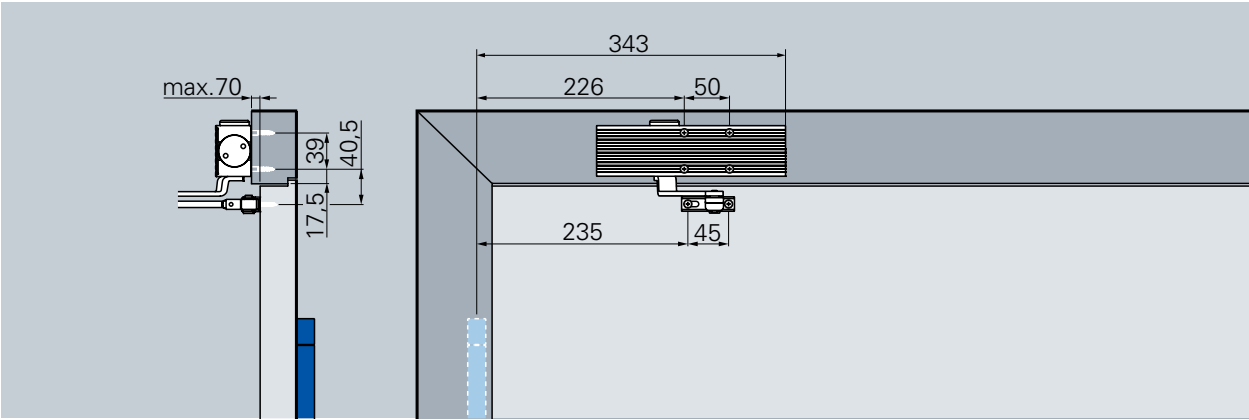
顶部安装, 铰链背侧 (EN 3)
