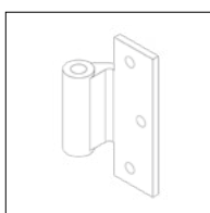
门框件
