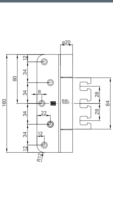
产品尺寸图
