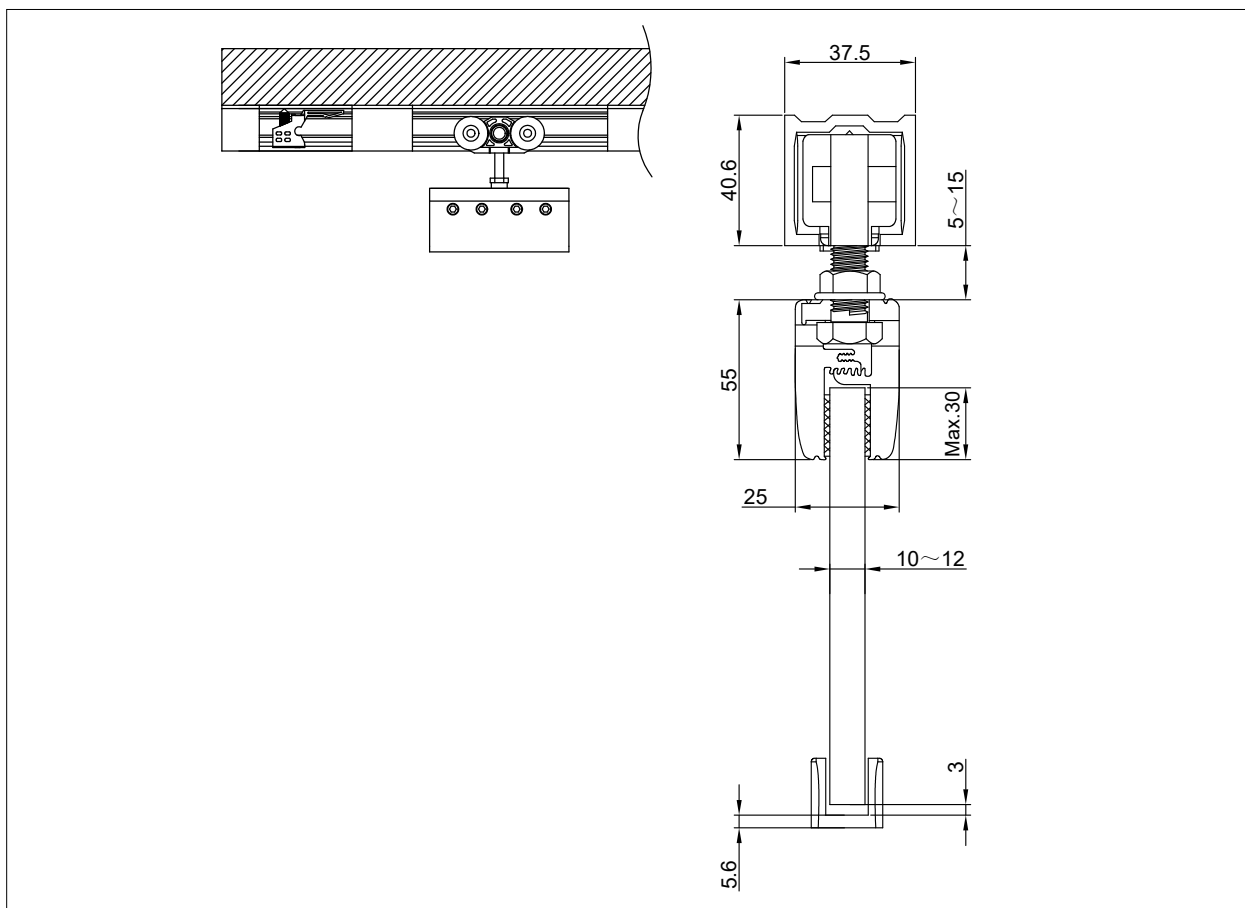
HR SL 120-G 玻璃推拉门示意图
