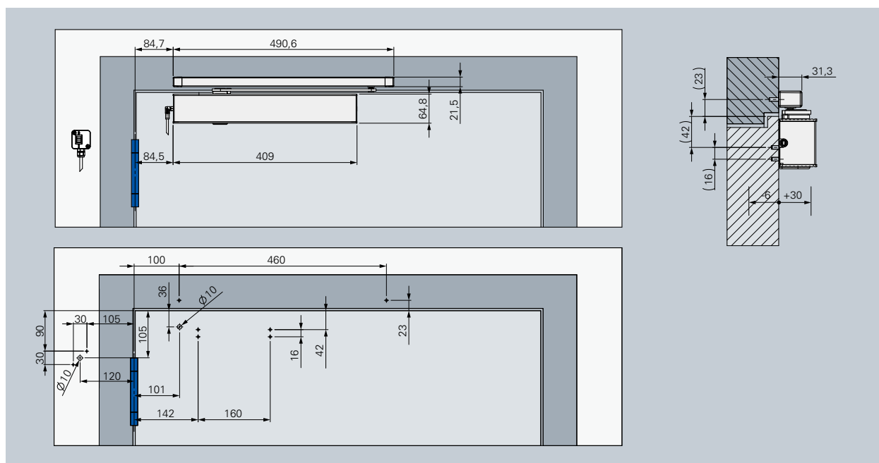
标准安装，铰链侧，DIN -L - ECO FTS III
