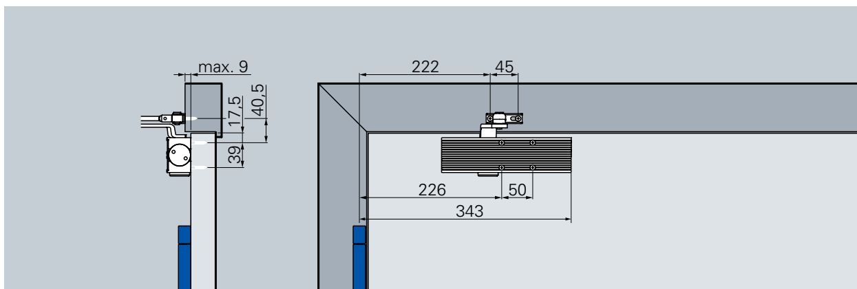
标准安装, 铰链侧 (EN 5)
