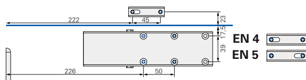
关门力度级别EN 4/5
