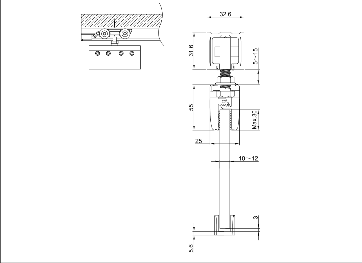
HR SL 80-G 玻璃推拉门示意图
