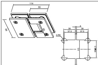
SH06 180°玻璃对玻璃浴室门夹
