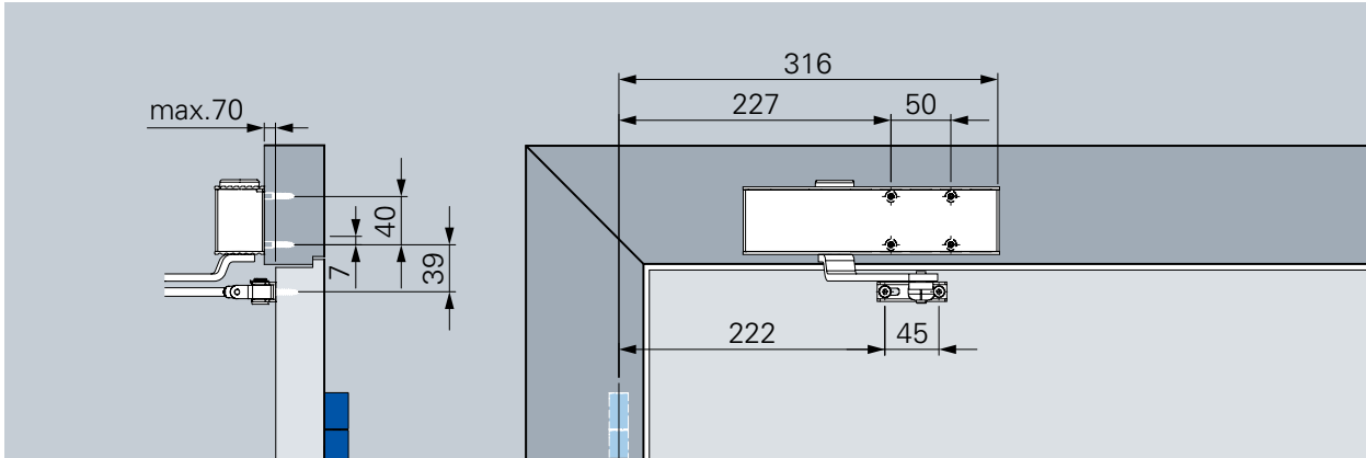
顶部安装, 铰链背侧 (EN 3), 带安装版
