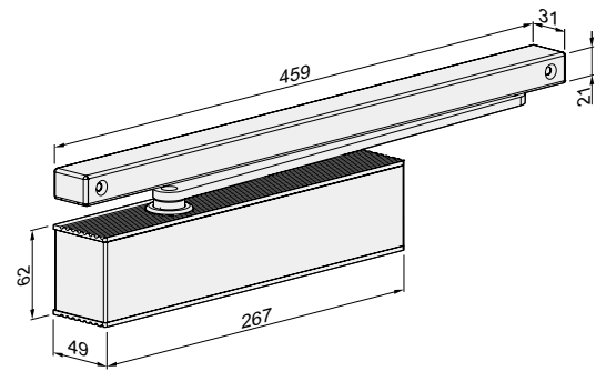
尺寸: TS-62 (2 - 5)
