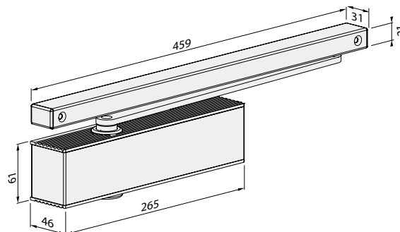
尺寸: TS-51
