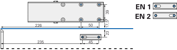
关门力度级别EN 1/2
