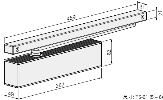
尺寸: TS-61 (5-6)
