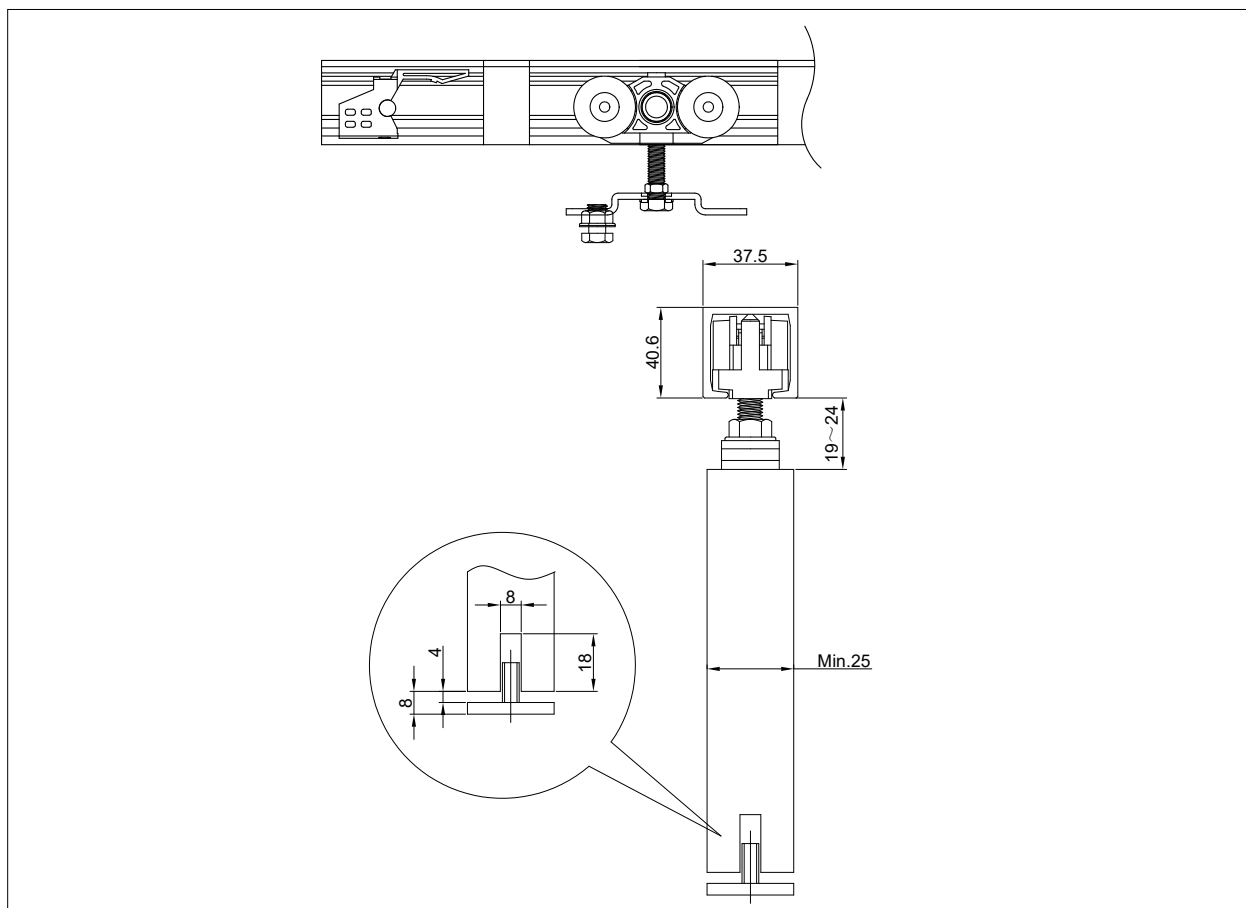
HR SL 100-W 木质推拉门示意图
