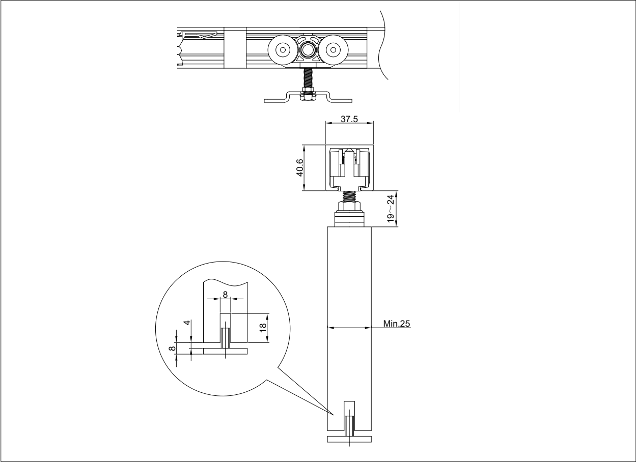
HR SL 60-W 木质推拉门示意图
