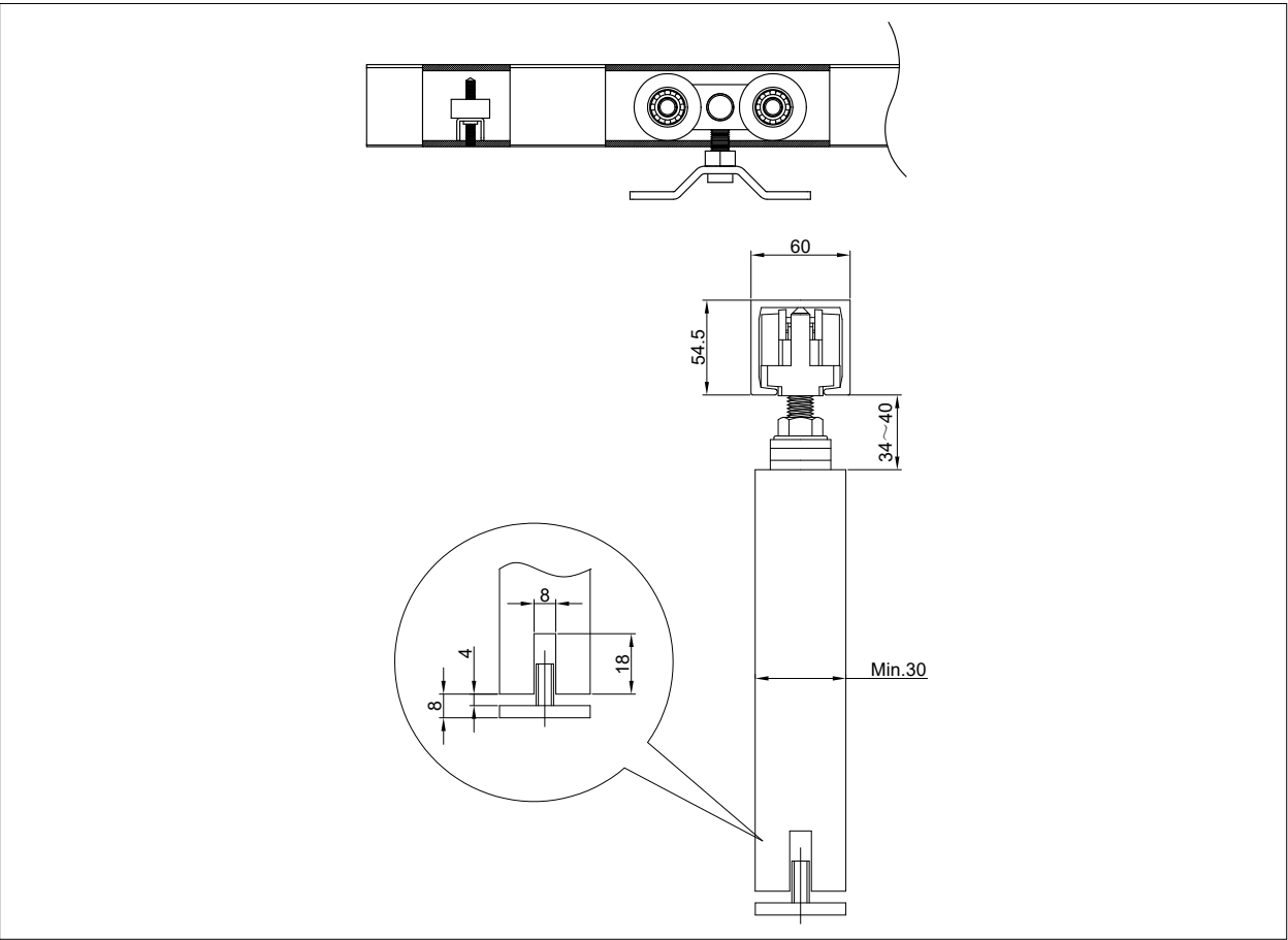
HR SL 250-W 木质推拉门示意图
